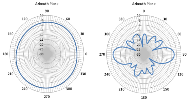
5900 MHz
